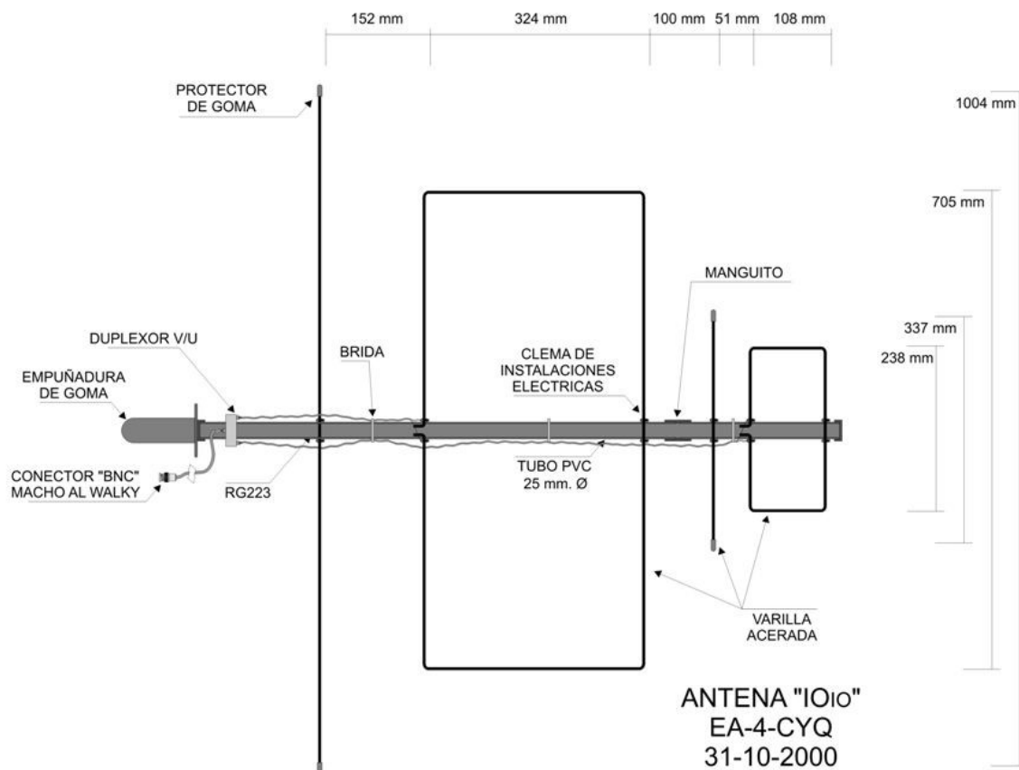
Esquema 1: Dimensiones constructivas de la antena IOio
